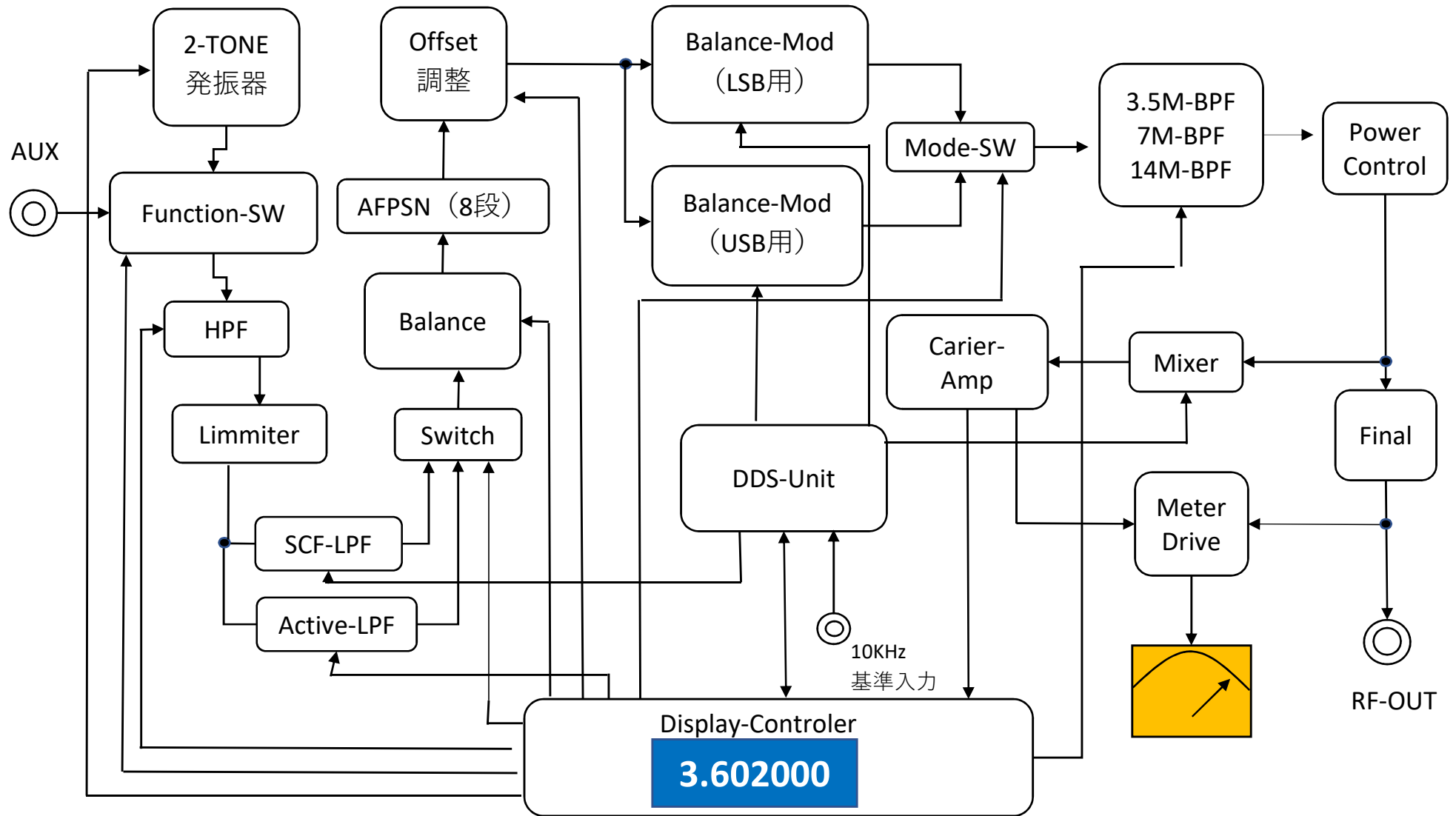
TX-Saturnブロック図
